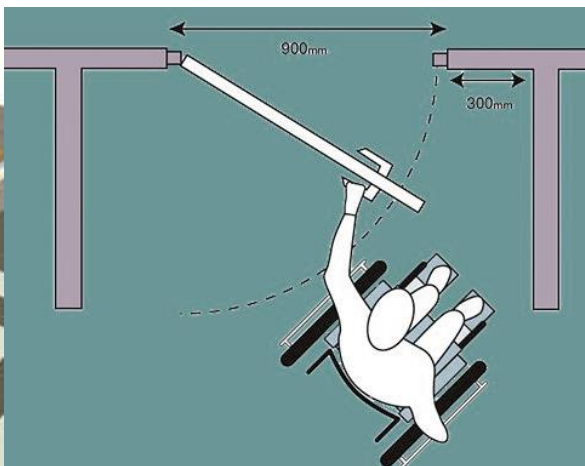
Figura 2: Situação ideal de abertura de porta para uma pessoa em cadeira de rodas.
